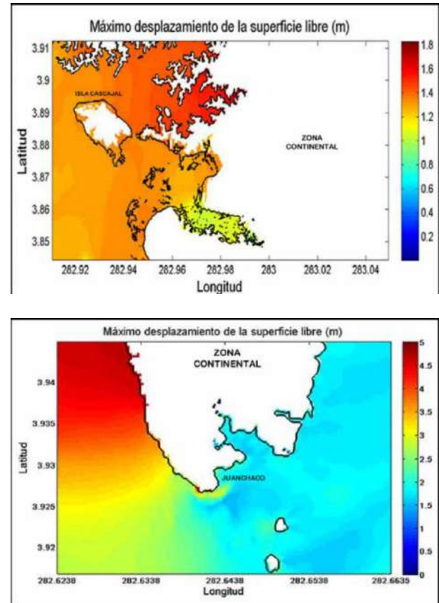
Figura 65. Propagación e inundación generada por el escenario sísmico E1. a) Casco Urbano de Buenaventura, b) Juanchaco.
