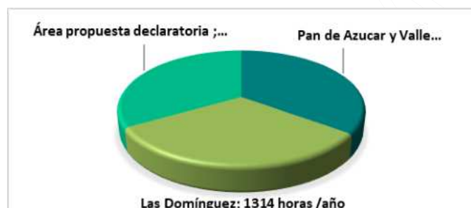
Gráfica 3. Brillo solar medio anual en el área propuesta para declaratoria.
