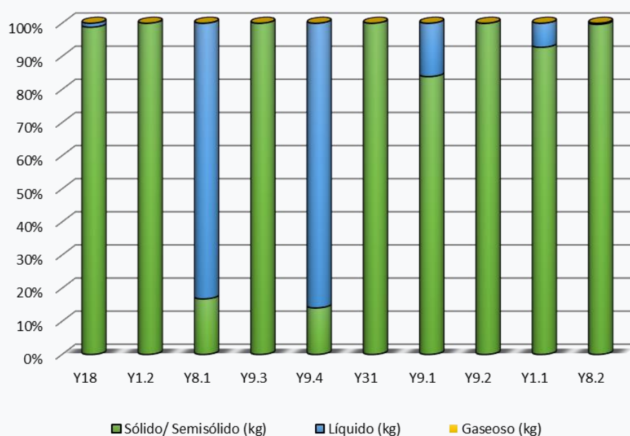
Gráfico 5. Aporte de generación (%) de los diez tipos de residuos peligrosos más generados en el periodo de balance 2024 por cada estado de la materia.
