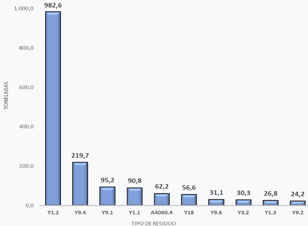
Gráfico 16. Cantidad reportada para los tipos de residuos peligrosos más gestionados a través de tratamiento en el periodo de balance 2024.
