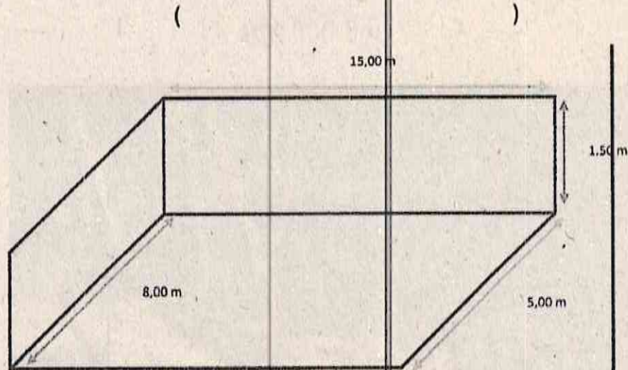
Figura 1. Esquema de las dimensiones de la excavación y explanación No. 2
